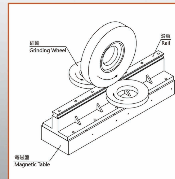
成型軌道三面同步研磨加工示意圖
